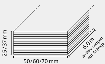
Dimensionen STEICO LVL RL Theaterlatten (mit Dickenkalibrierung)
