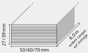
Dimensionen STEICO LVL RL Theaterlatten (ohne Dickenkalibrierung)
